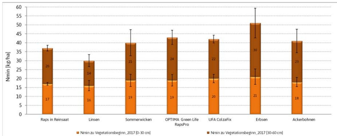
Abbildung 9: Mittelwerte und Standardabweichungen des Gehalts an Nitratstickstoff zu Vegetationsbeginn 2017 am Standort Scheppau bei einer Probenahmetiefe von 0-60 cm. Anzahl der Wiederholungen: n=4 (Bei Raps in Reinsaat: n=16).
