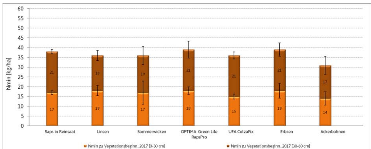
Abbildung 10: Mittelwerte und Standardabweichungen des Gehalts an Nitratstickstoff zu Vegetationsbeginn 2017 am Standort Klein Escherde bei einer Probenahmetiefe von 0-60 cm. Anzahl der Wiederholungen: n=4 (Bei Raps in Reinsaat: n=16).
