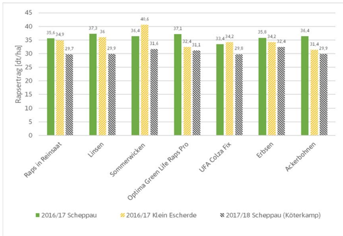
Abbildung 13: Rapsertträge in dt/ha nach Art der Begleitpflanzen an den Standorten Scheppau und Klein Escherde in beiden Versuchsjahren. Bei der Variante Raps in Reinsaat ist der Mittelwert der Parzellen angegeben (2016/17: n=4; 2017/18: n=3).
