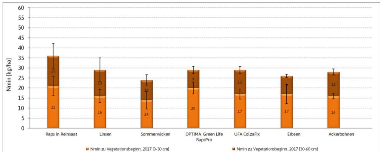
Abbildung 12: Mittelwerte und Standardabweichungen des Gehalts an Nitratstickstoff zu Vegetationsbeginn 2018 am Standort Scheppau (Ackern) bei einer Probenahmetiefe von 0-60 cm. Anzahl der Wiederholungen: n=4 (Bei Raps in Reinsaat: n=16).
