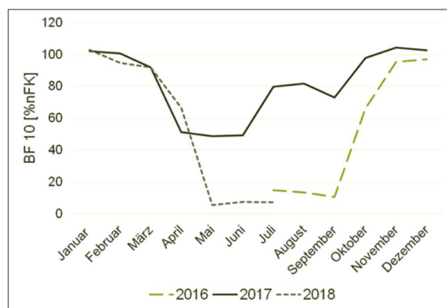
Abbildung 4: Bodenfeuchteverlauf 2016-2018
