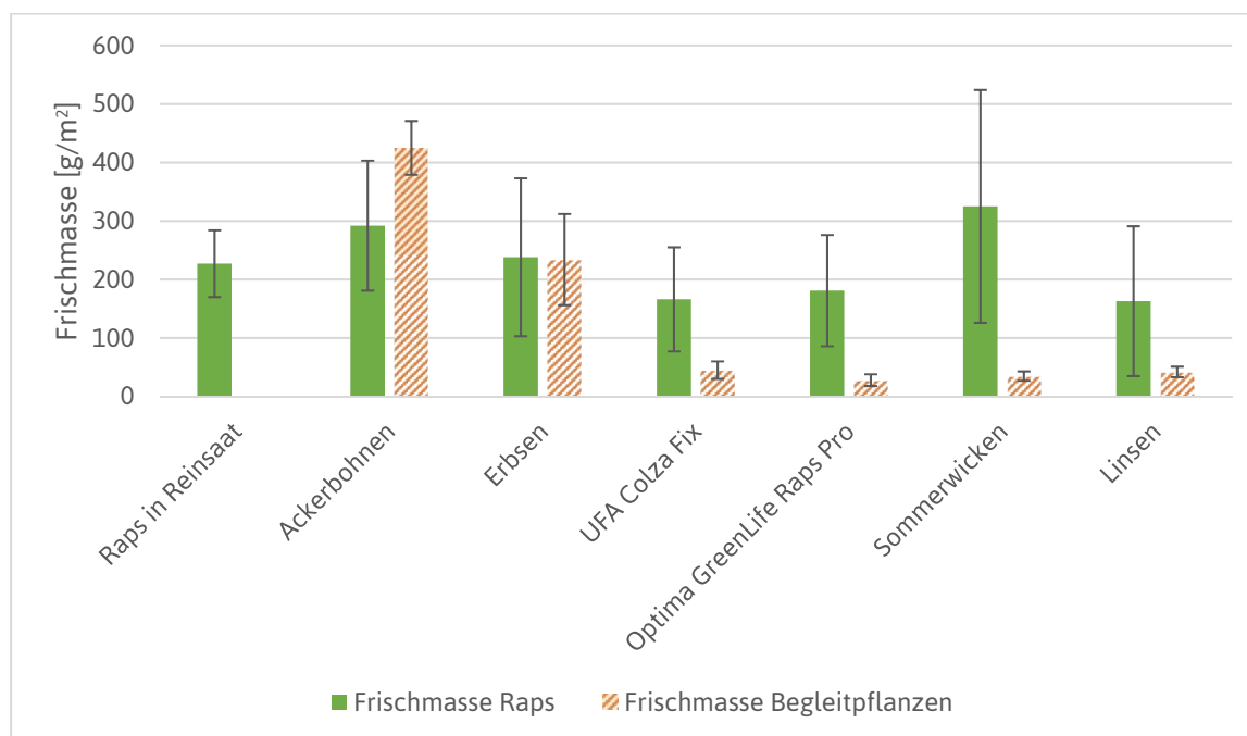
Abbildung 7: Oberirdische Frischmasse zum Vegetationsende von Raps und Begleitpflanzen in g/m². Versuchsjahr 2017/18 am Standort Scheppau auf dem Schlag Kötterkamp. Mittelwerte und Standardabweichung (n=4; Variante Raps in Reinsaat: n=16).
