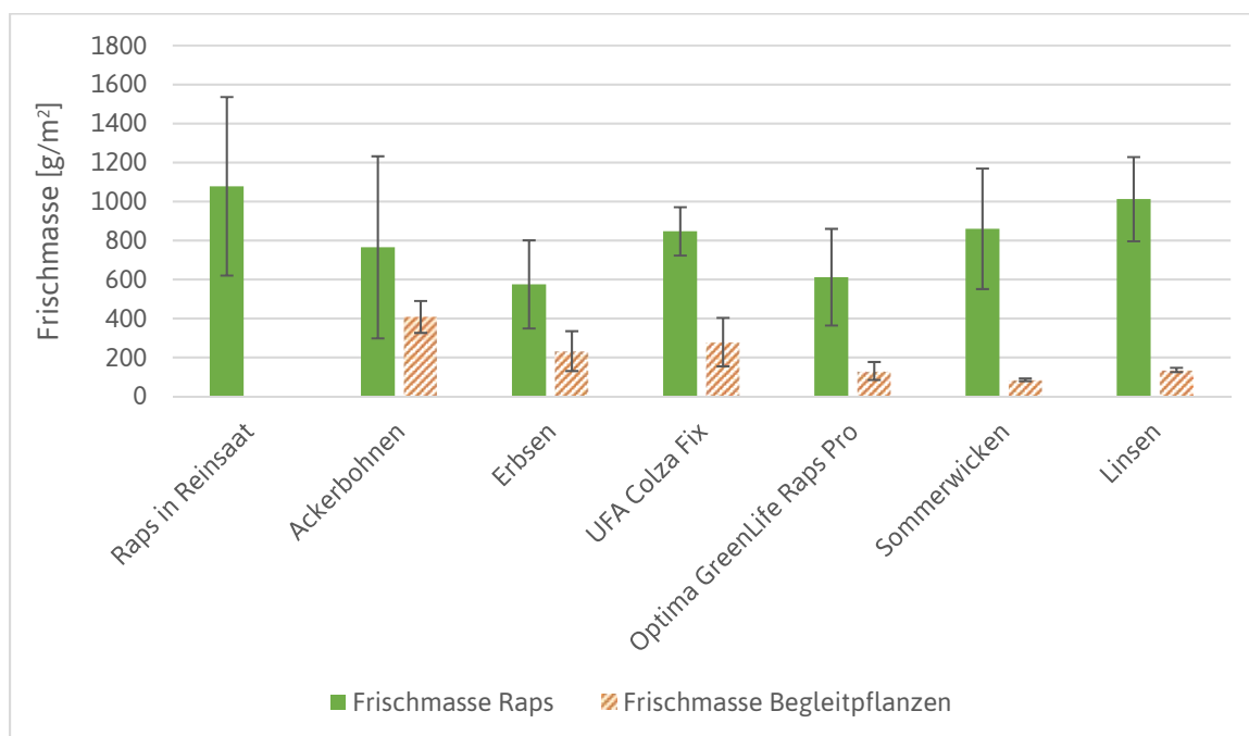
Abbildung 5: Oberirdische Frischmasse zum Vegetationsende von Raps und Begleitpflanzen in g/m². Versuchsjahr 2016/17 am Standort Scheppau. Mittelwerte und Standardabweichung (n=4).
