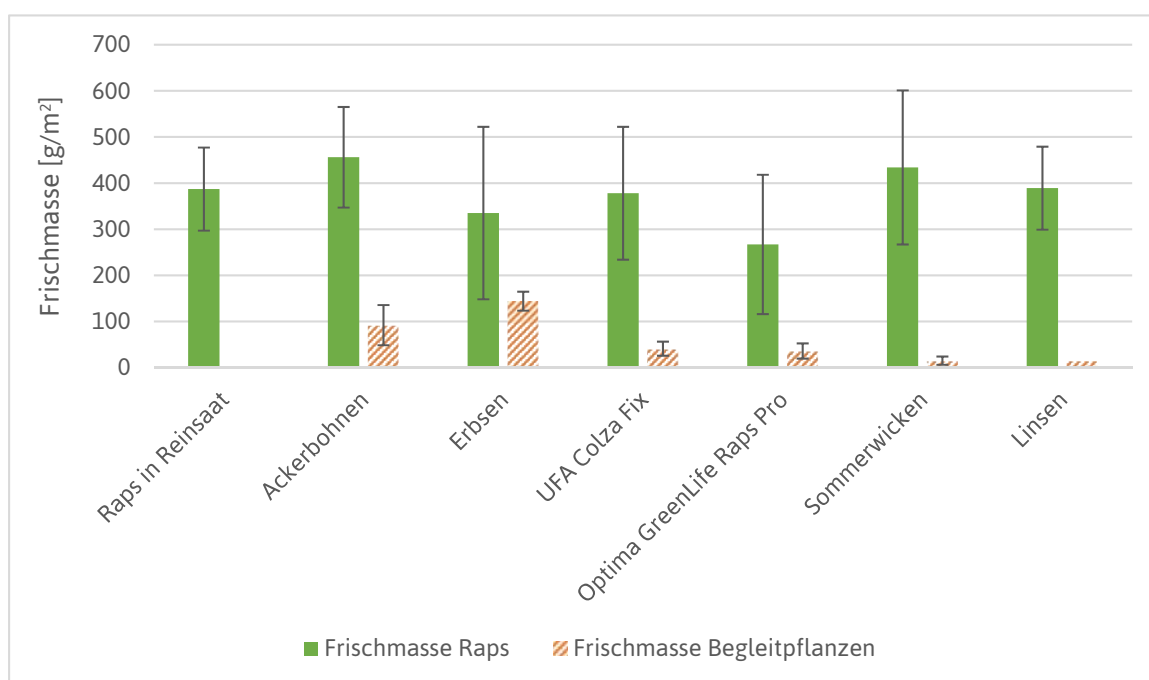
Abbildung 6: Oberirdische Frischmasse zum Vegetationsende von Raps und Begleitpflanzen in g/m². Versuchsjahr 2016/17 am Standort Klein Escherde. Mittelwerte und Standardabweichung (n=4).
