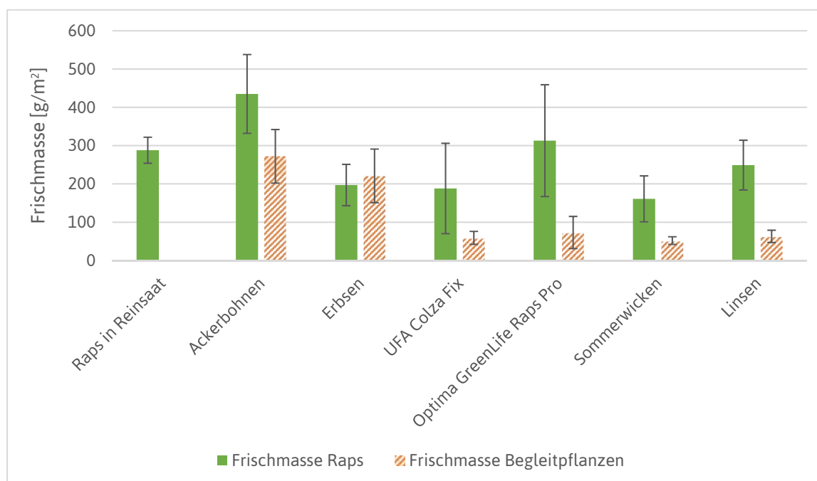
Abbildung 8: Oberirdische Frischmasse zum Vegetationsende von Raps und Begleitpflanzen in g/m². Versuchsjahr 2017/18 am Standort Scheppau auf dem Schlag Ackern. Mittelwerte und Standardabweichung (n=4; Variante Raps in Reinsaat: n=16).
