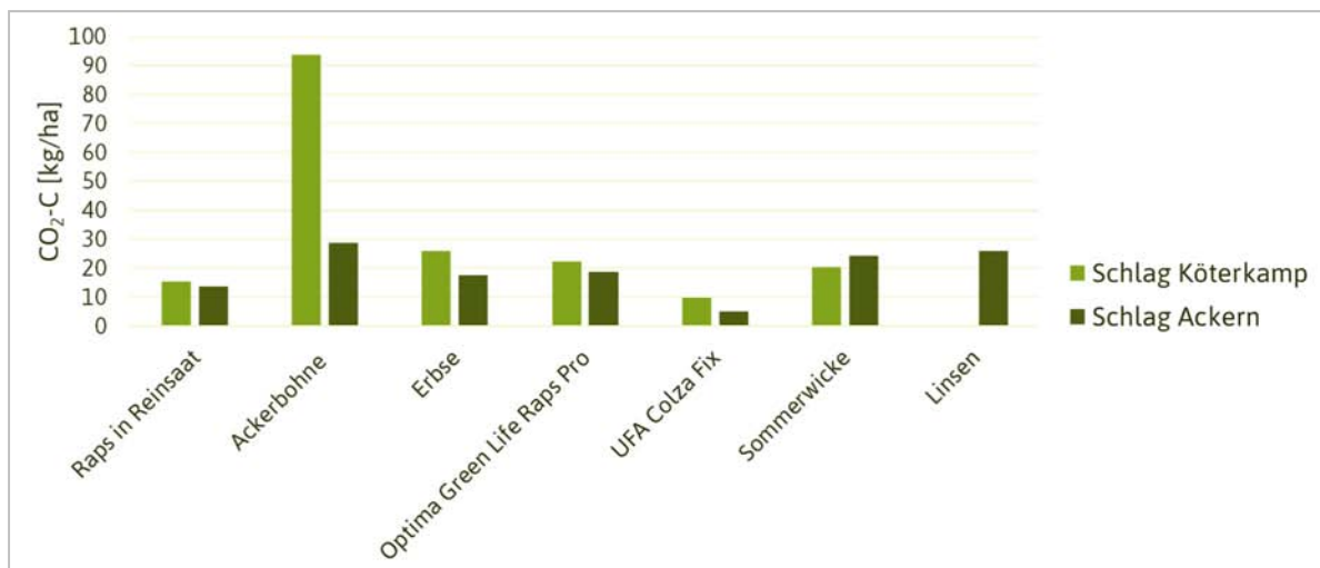
Abbildung 14: Bestimmung des CO 2 -C über den Soilvita Test
